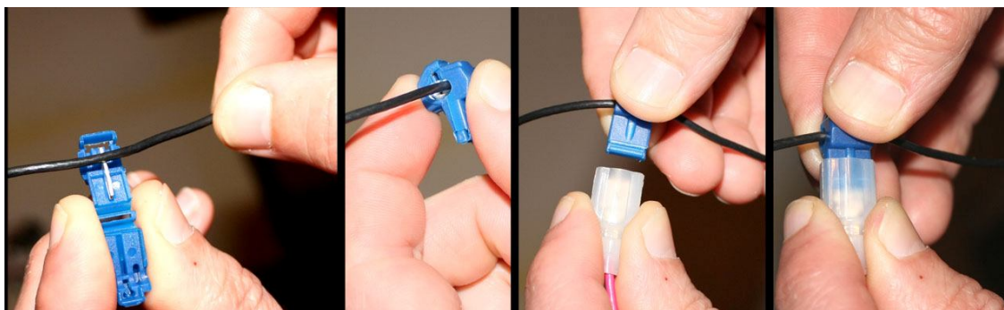
Рисунок 3.3. Методика подключения проводов при помощи быстрых соединителей.
