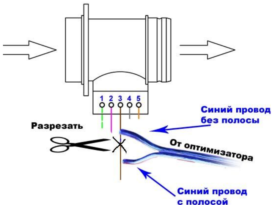
Рисунок 3.4. схема подключения датчика массового расхода воздуха для автомобилей ВАЗ, Daewoo (цоколёвка датчика может отличаться).
