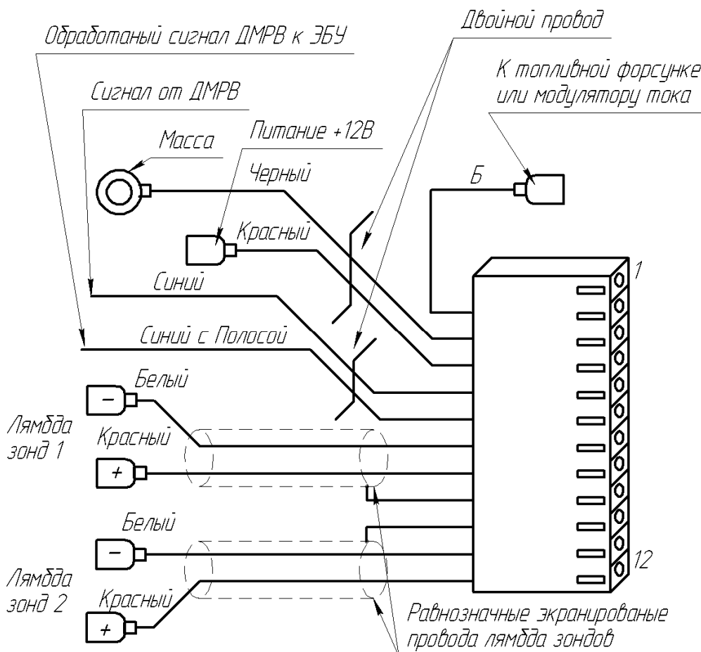
Рисунок 3.2. Назначение проводов.
